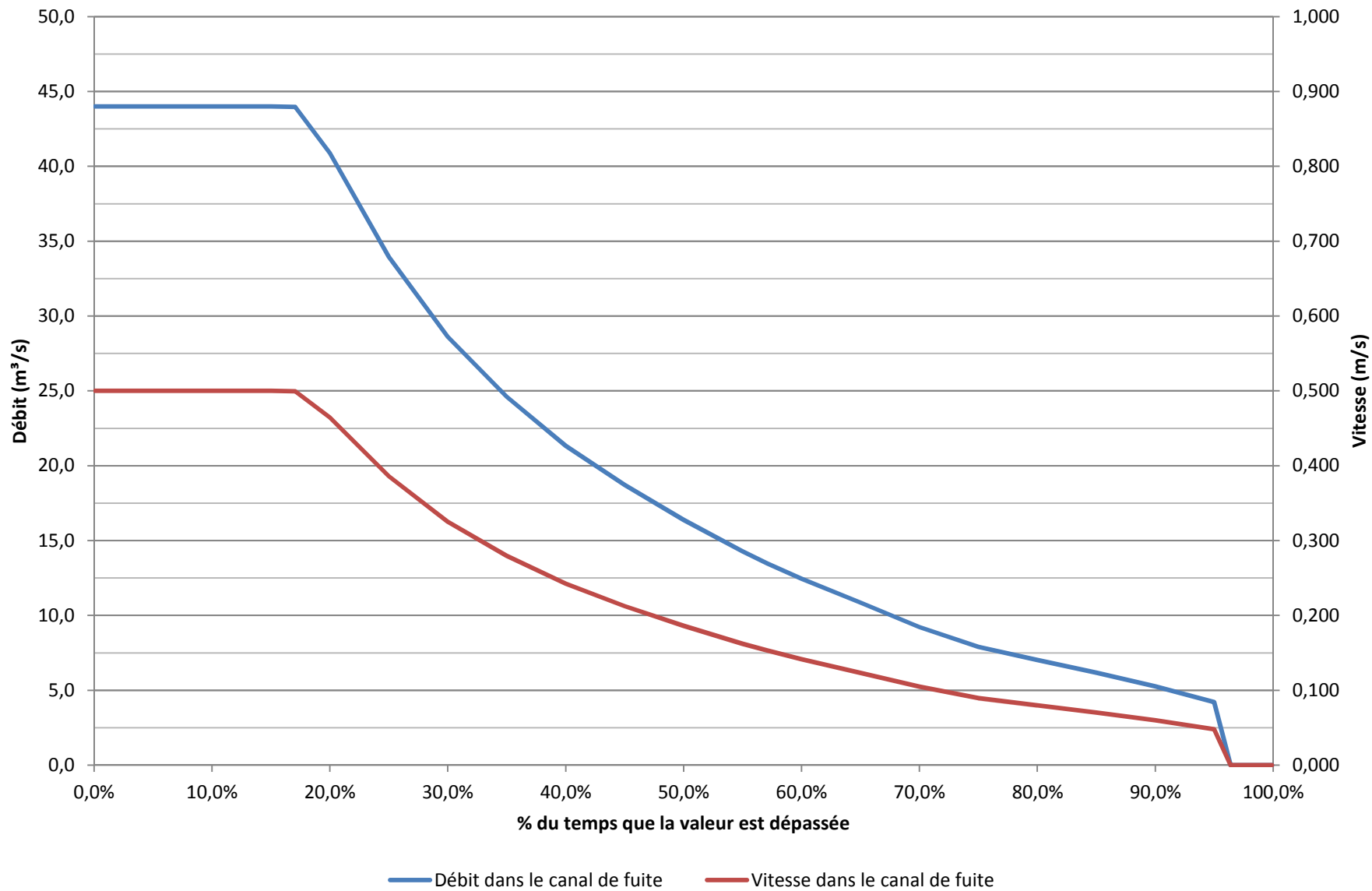
Figure A-3 : Représentation temporelle des débits et vitesses rencontrés dans le canal de fuite
